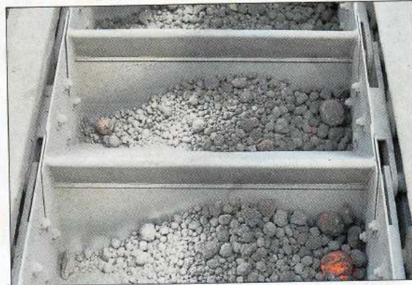
Der Schotter wird in einer Kugelmühle mit Ofenabgas getrocknet und zu Rohmehl gemahlen, das auf bis zu 1450 Grad erhitzt und in den hier auf dem Bild abgebildeten Zementklinker umgewandelt wird.
